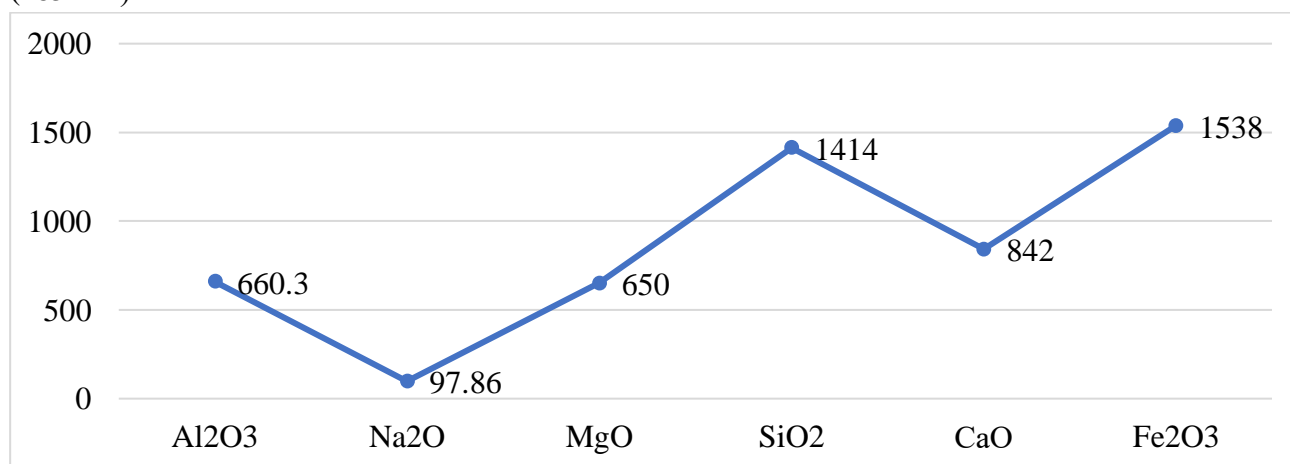
Расми 1. Ҳарорати моеъшавии элементҳо (на пайвастагӣҳо), ^{\circ}C
