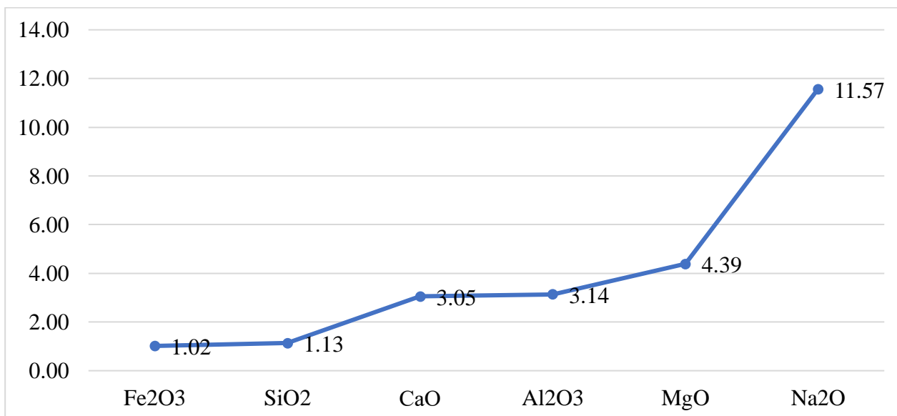
Расми 3. Ҳарорати моеъшавии пайвастагиҳо нисбат ба элементҳо
