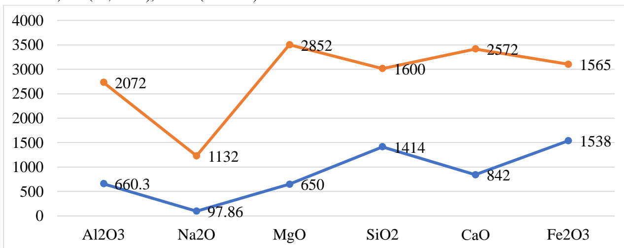
Расми 2. Ҳарорати моеъшавии элементҳо ва пайвастагиҳои онҳо, °C
